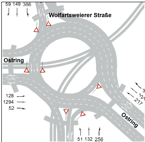
Abb 6. Prognostizierte Verkehrsbelastungen und Vorfahrtregelung für Kreisverkehr „Ostring“
